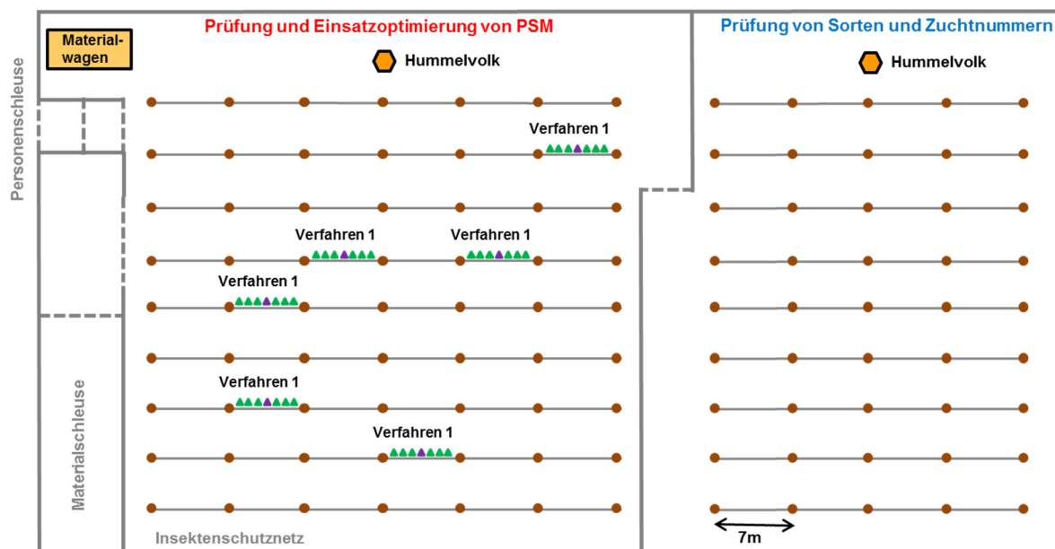
Abbildung 1: Parzellenplan BR 53.
